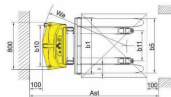
CDD10B-III CDD15B-III
