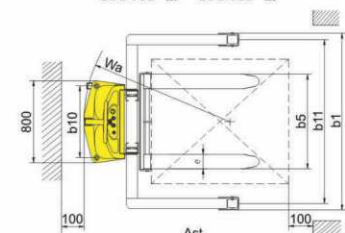
CTD10B-III CTD15B-III
